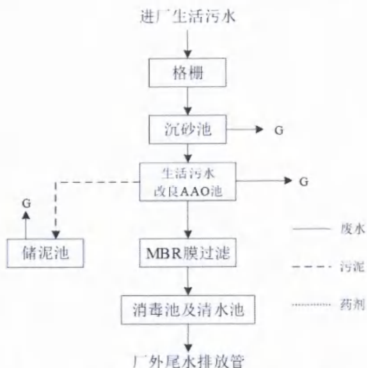
图 4-2 吴江市盛泽水处理发展有限公司（南部工业区综合污水处理厂）工艺图
