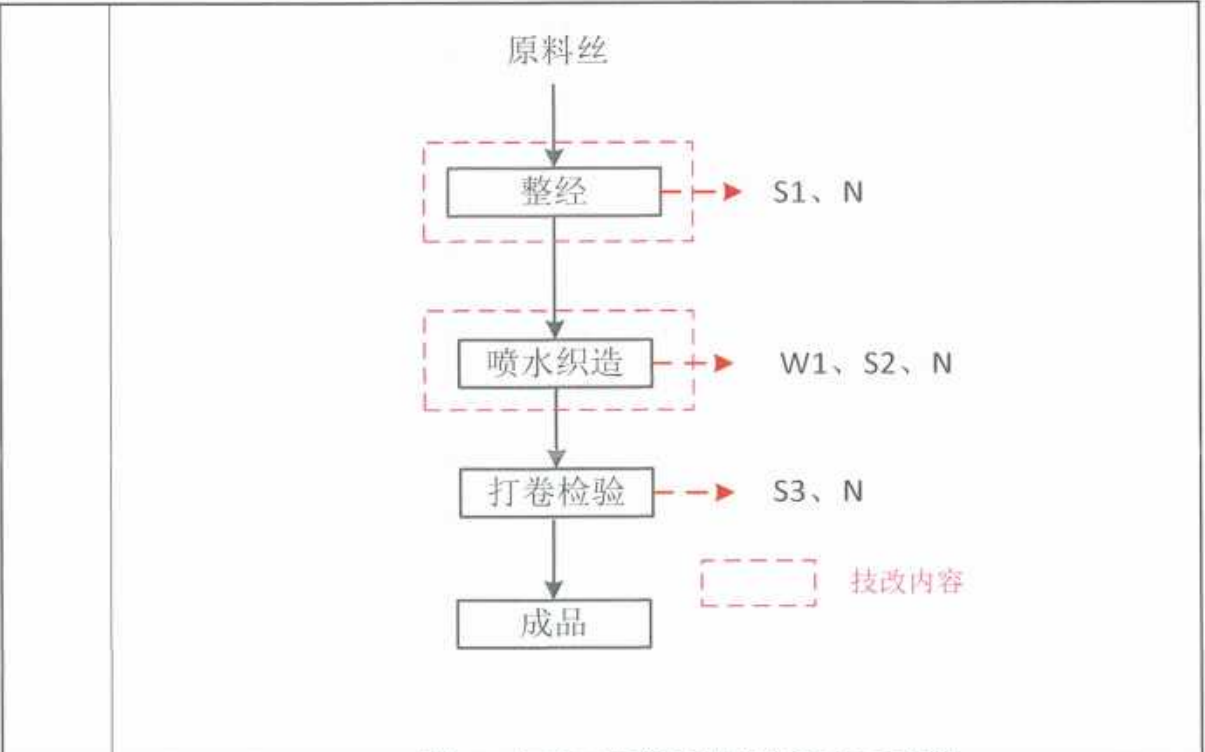
图 2-3 生产工艺流程及产污环节示意图
