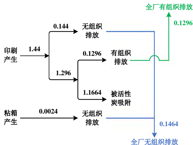
图 2-2 本项目 VOCs 平衡图（单位：t/a）
