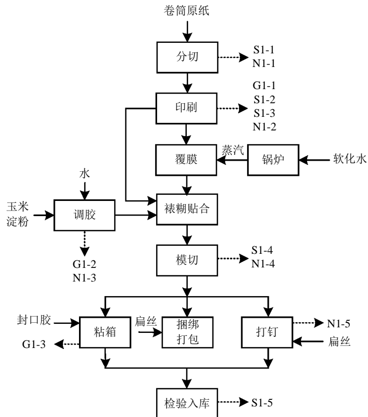
图 2-3 纸箱生产工艺流程及产污环节
