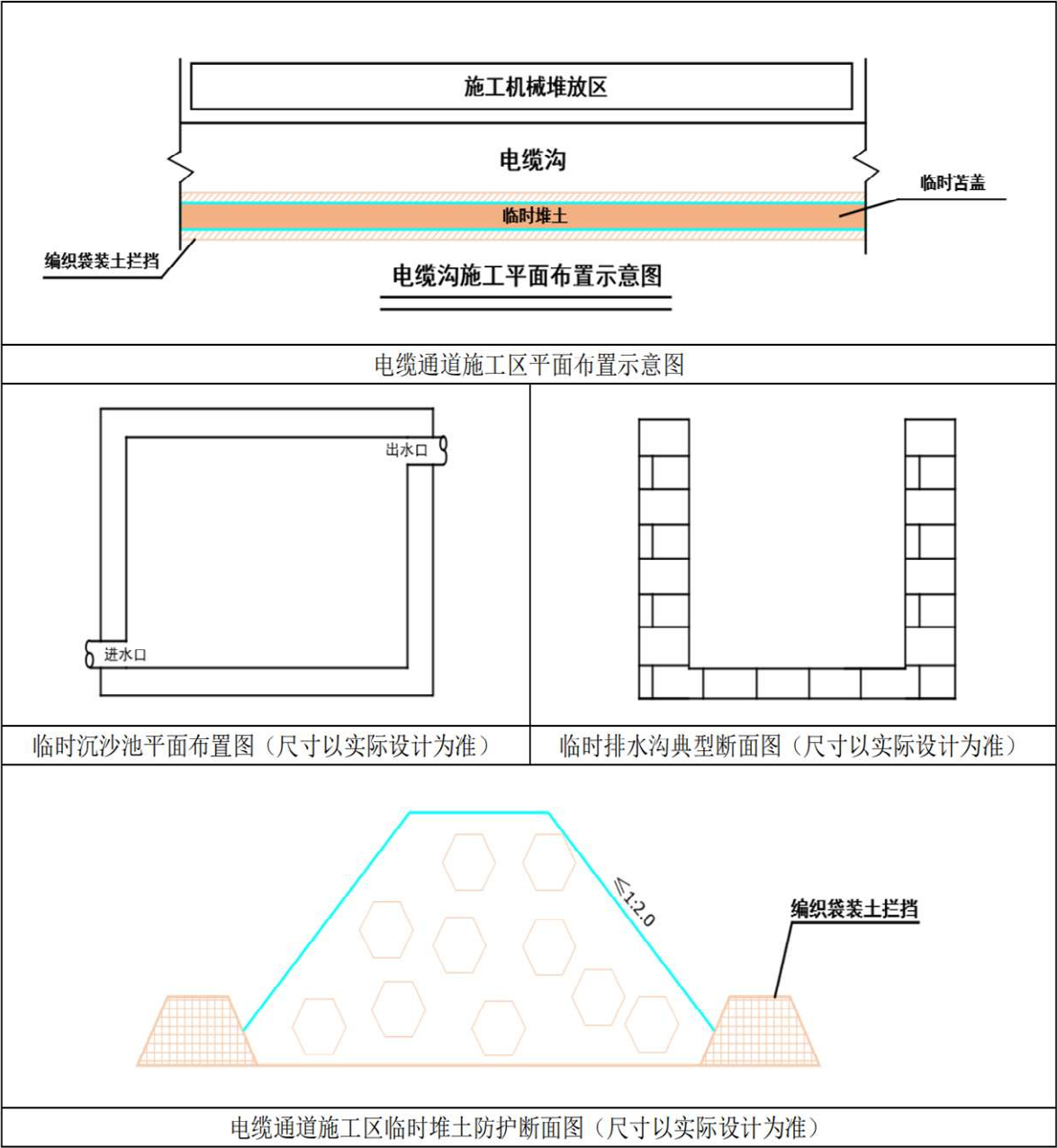
附图 7 本项目典型环保设施设计图（电缆通道施工）
