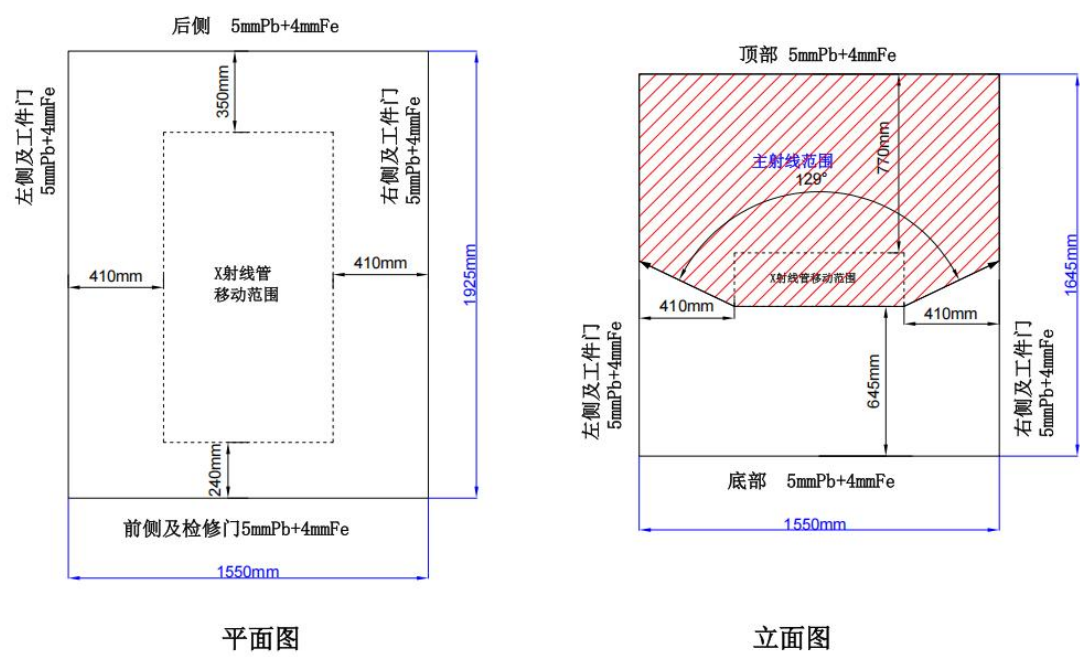
图 11-1 本项目工业 CT 检测装置辐射源点到各侧屏蔽体最近距离示意图
