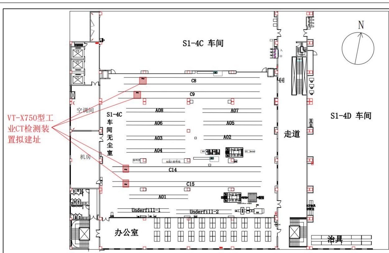
图 8-1 S1-4C 车间无尘室 4 台 OmronVT-X750 型工业 CT 检测装置位置示意图 本项目工业 CT 检测装置拟建场址和周边环境现状见图 8-2。
