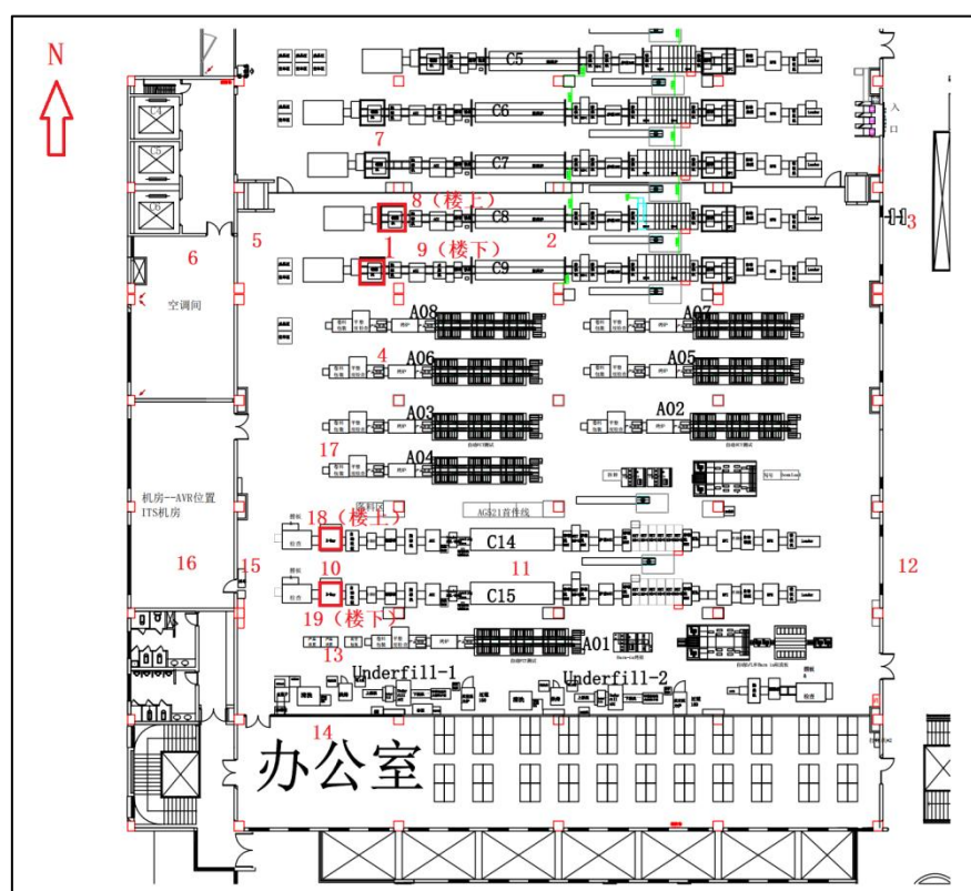
图 8-3 S1-4C 车间无尘室 C8、C9、C14、C15 号生产线 OmronVT-X750 型工业 CT 检测装置拟建场址周围环境 \gamma 辐射剂量率监测点位示意图
