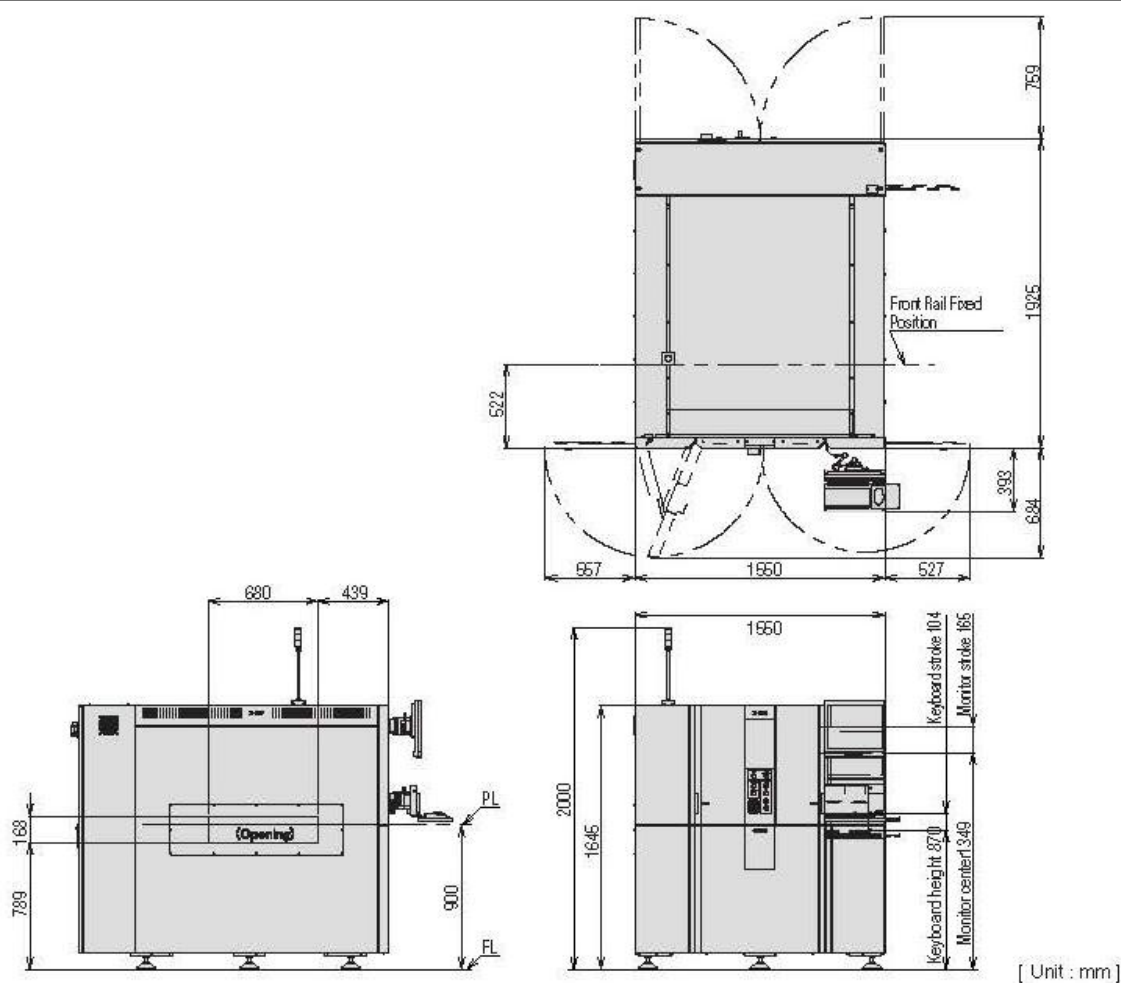
图 9-2 OmronVT-X750 型工业 CT 检测装置外观尺寸图（单位：mm）
