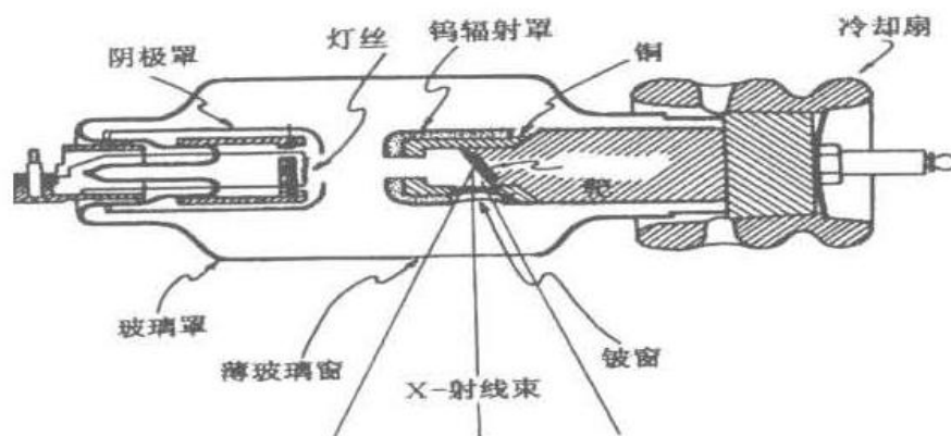
图 9-3 典型的 X 射线管结构图
