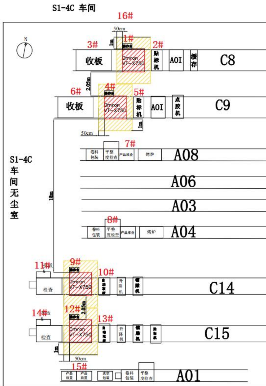
图 11-3 本项目估算点位示意图
