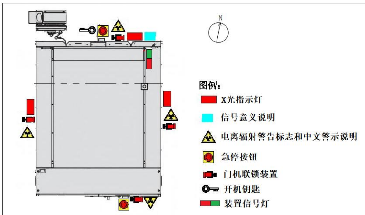
图 10-2 OmronVT-X750 型工业 CT 检测装置安全措施示意图
