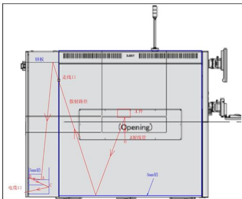
图 11-2 电缆口防护罩结构散射示意图
