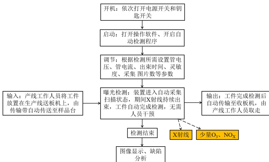
图 9-4 本项目射线装置工艺流程及产污环节分析示意图
