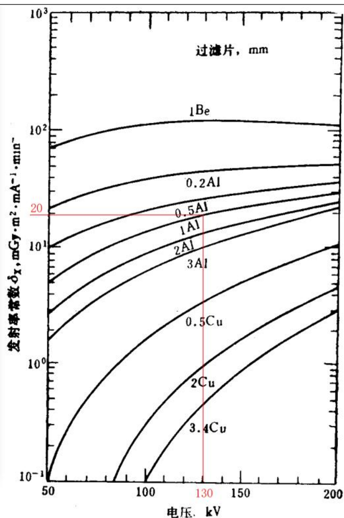
图 9-5 有用线束辐射输出量取值图
