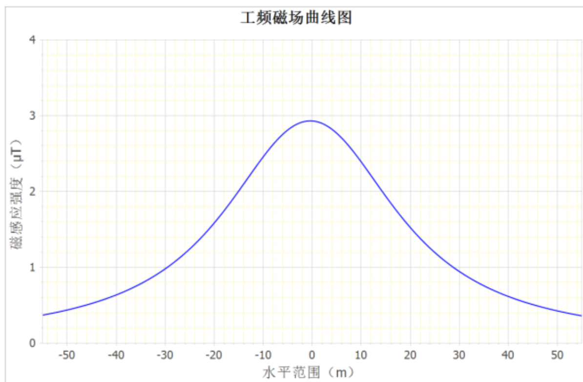
图 3-2 110kV 湖阳/新阳线新建段架空线路下工频磁场随距离变化趋势图
