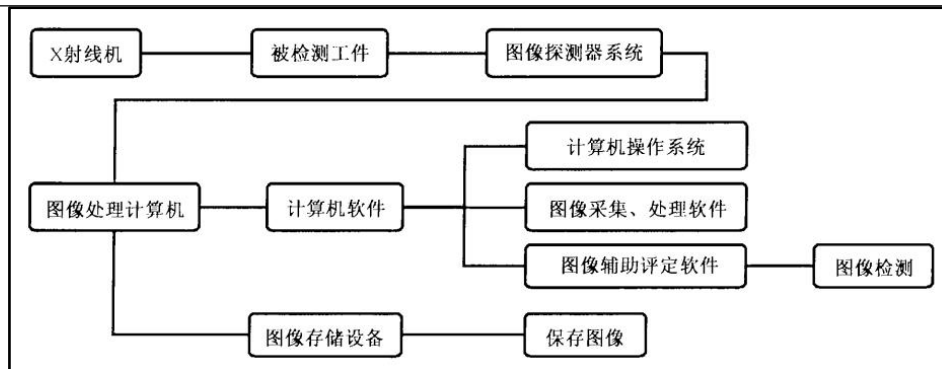
图 9-3 典型 X 射线实时成像工作原理图
