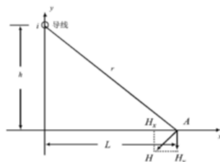
图 3-4 磁场向量图
