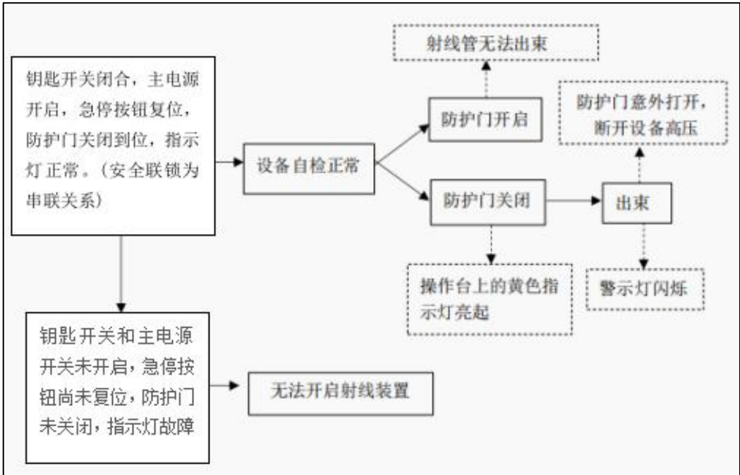
图10-2 联锁逻辑图
