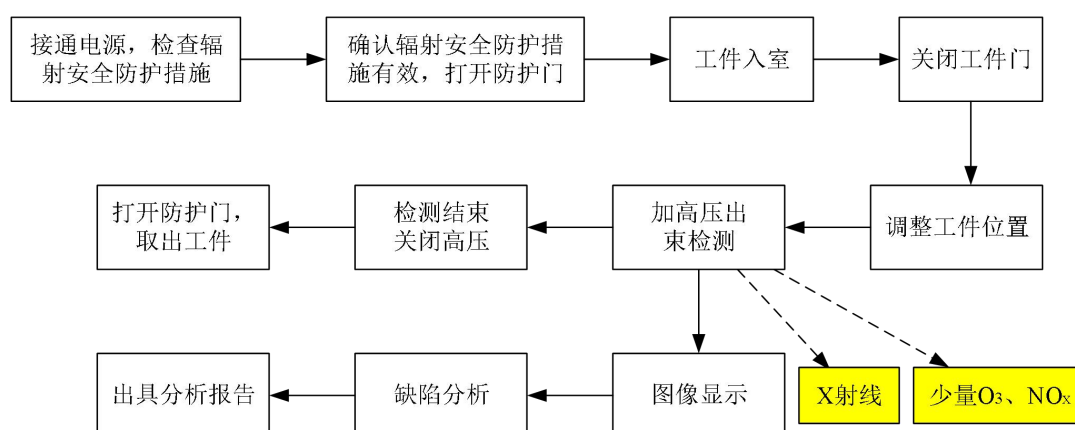
图9-7 工业探伤装置工作流程及产污环节示意图
