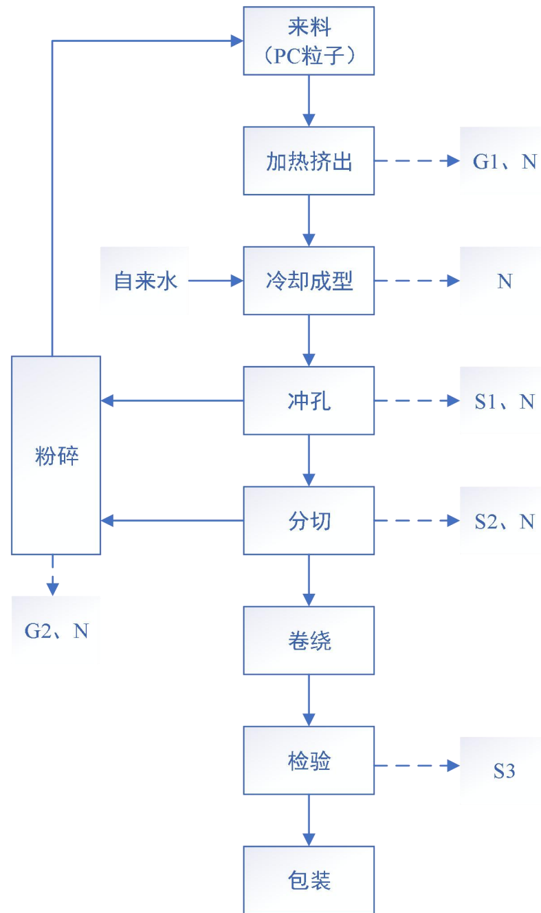
图2-2 载带工艺流程图(原料为PC塑料粒子)
