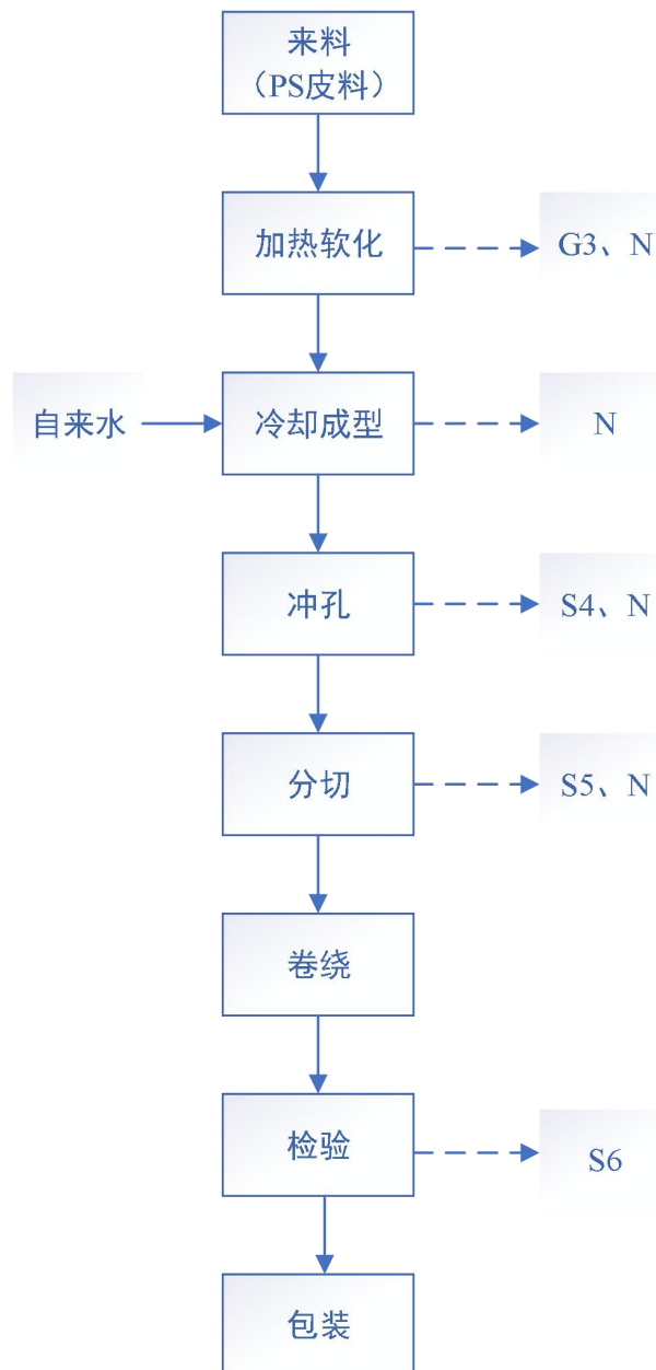
图2-3 载带工艺流程图(原料为PS皮料)
