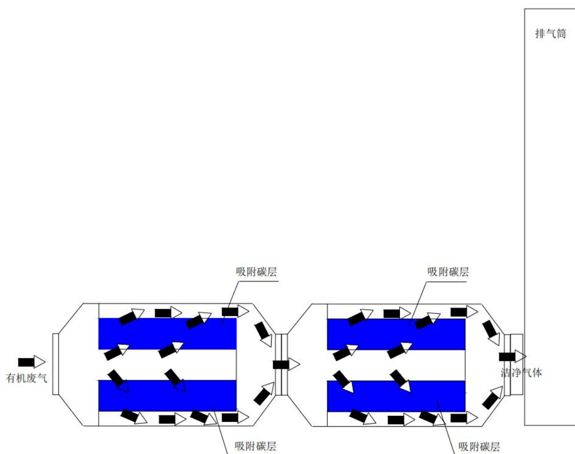
图 4-1 有机废气进两级活性炭箱走向示意图
