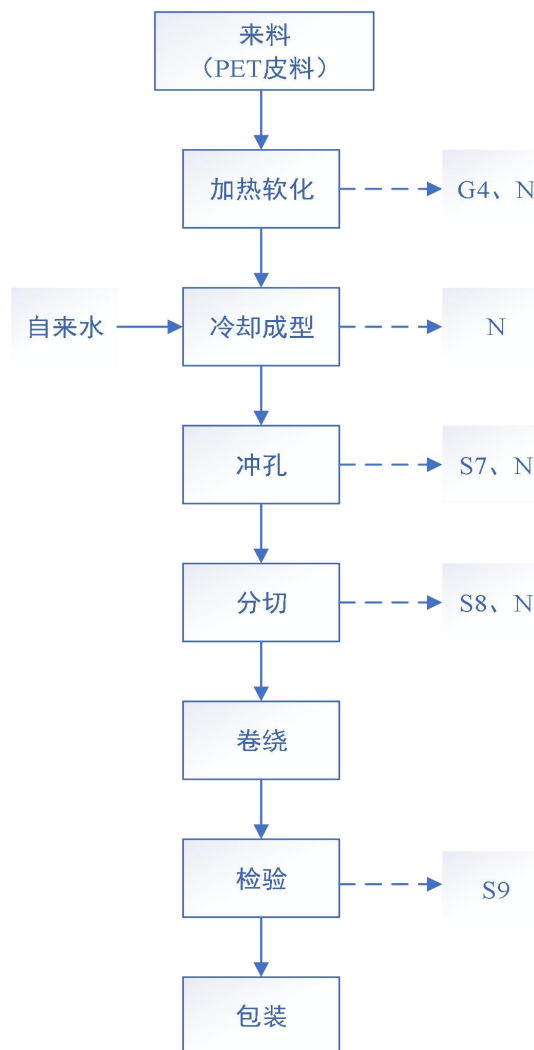
图2-4 载带工艺流程图(原料为PET皮料)
