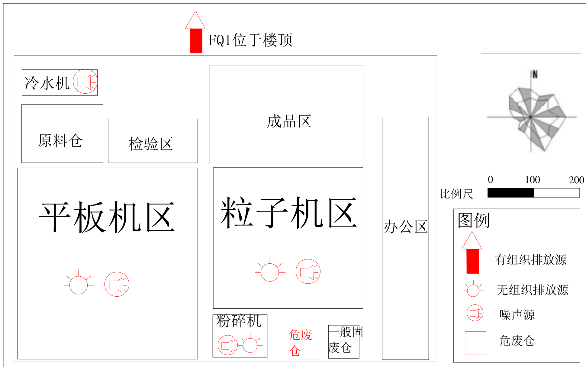
附图2 厂区平面布置图
